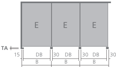
Einzelanlage für 2 Pkw
